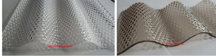
PC-Wellplatten, Wabenstruktur
